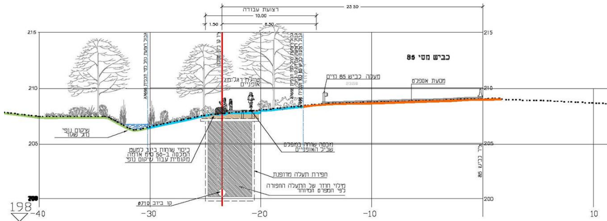
איור 20: חתך אופייני, טיילת לאורך כביש 86 95 .
